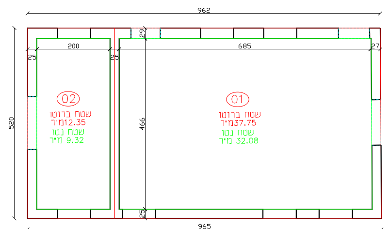
קומת קרקע קנ"ם: 1:100
