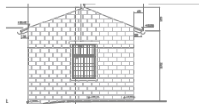
חזית מערבית
