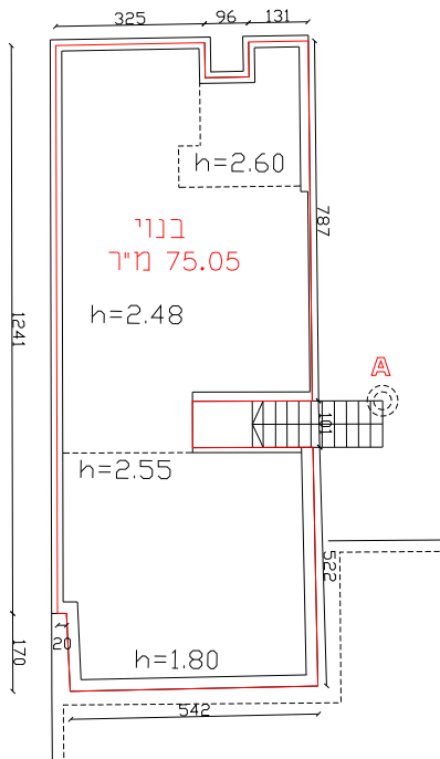
קומת גלריה
