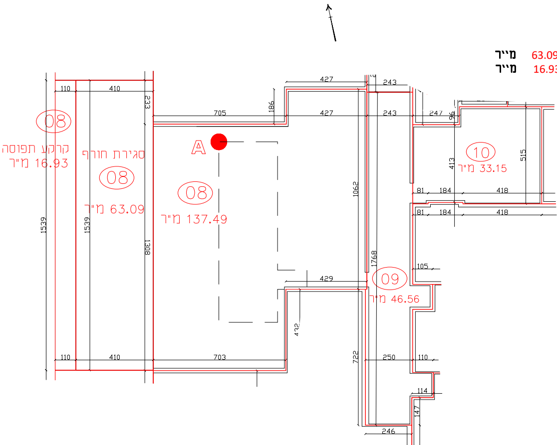
קומת קרקע
