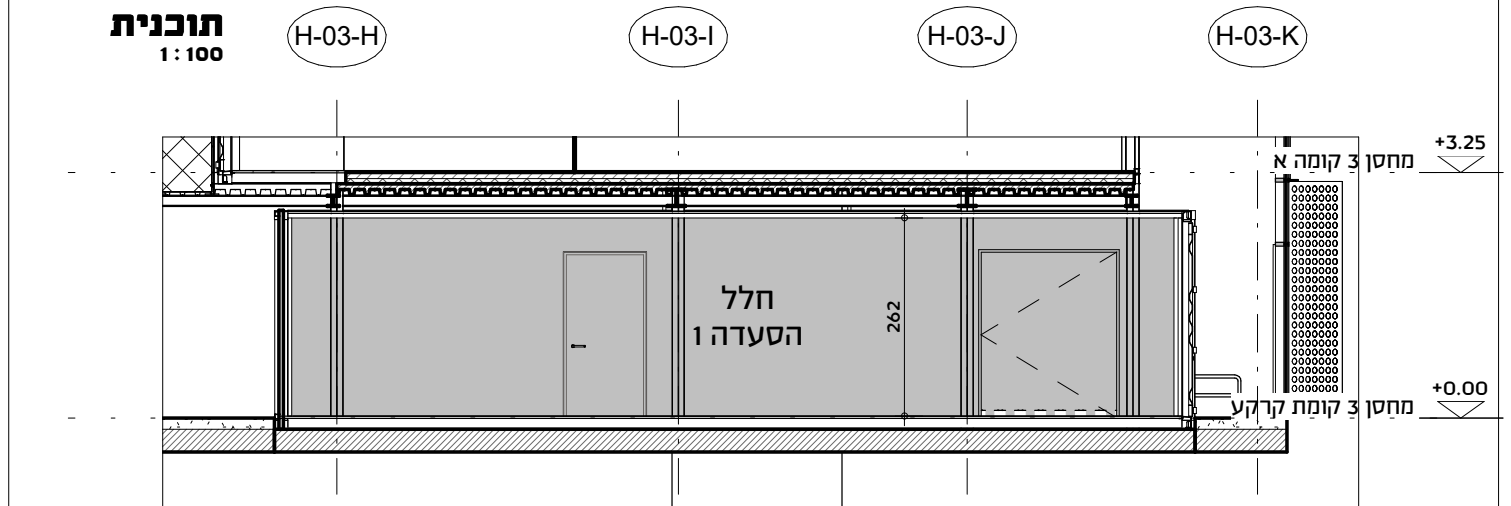
חתך 1 : 100
