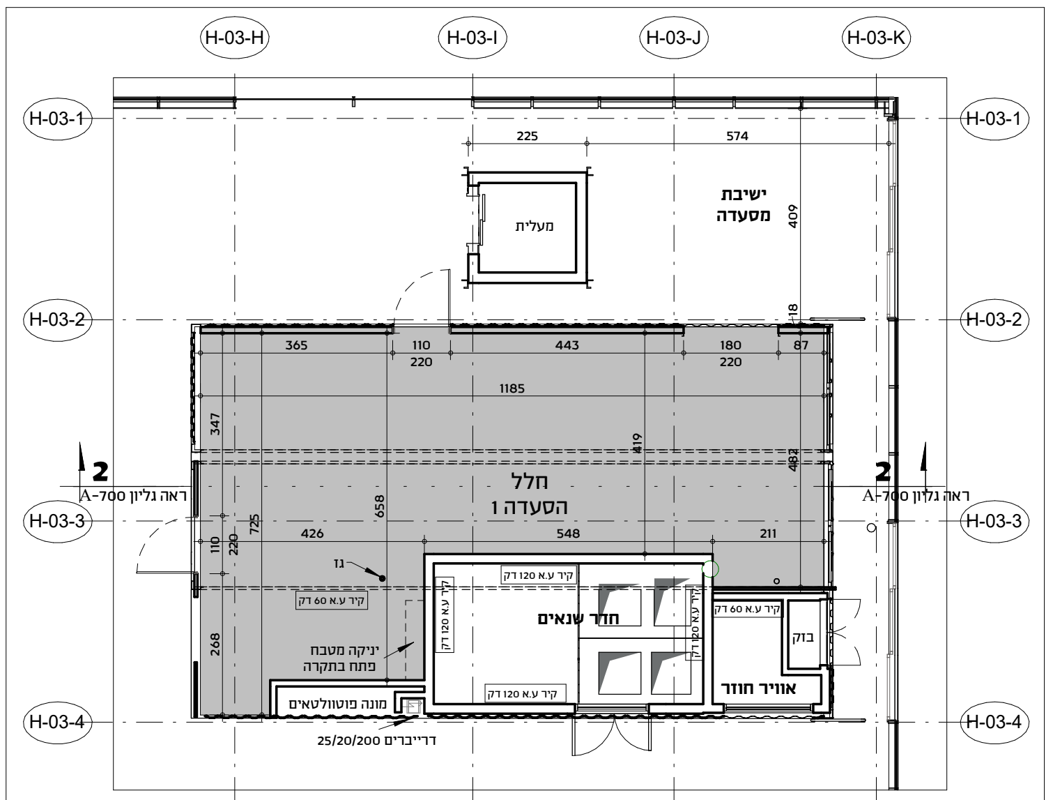
תוכנית 1 : 100
