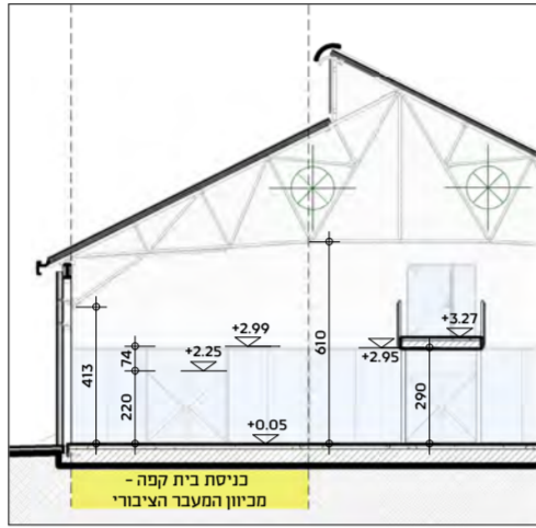
חזית כניסה לבית הקפה מהמעבר הציבורי 1 : 250
