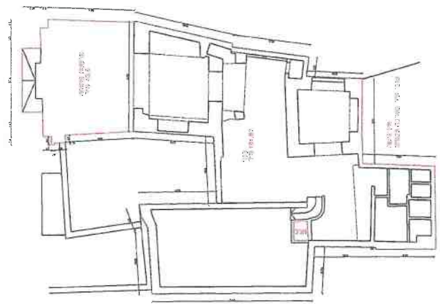
קומת קרקע
