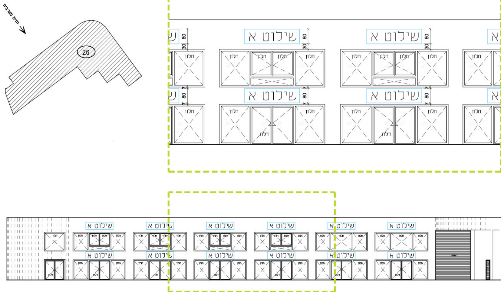
מבנה 26 חזית מערבית
