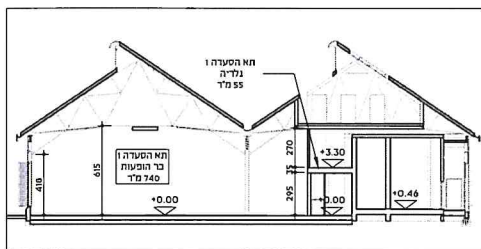
7 חתך רוחב דרך הגלריה 1: 250
