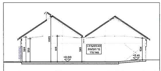
5 חתך רוחב מזרח מערב 1: 250
