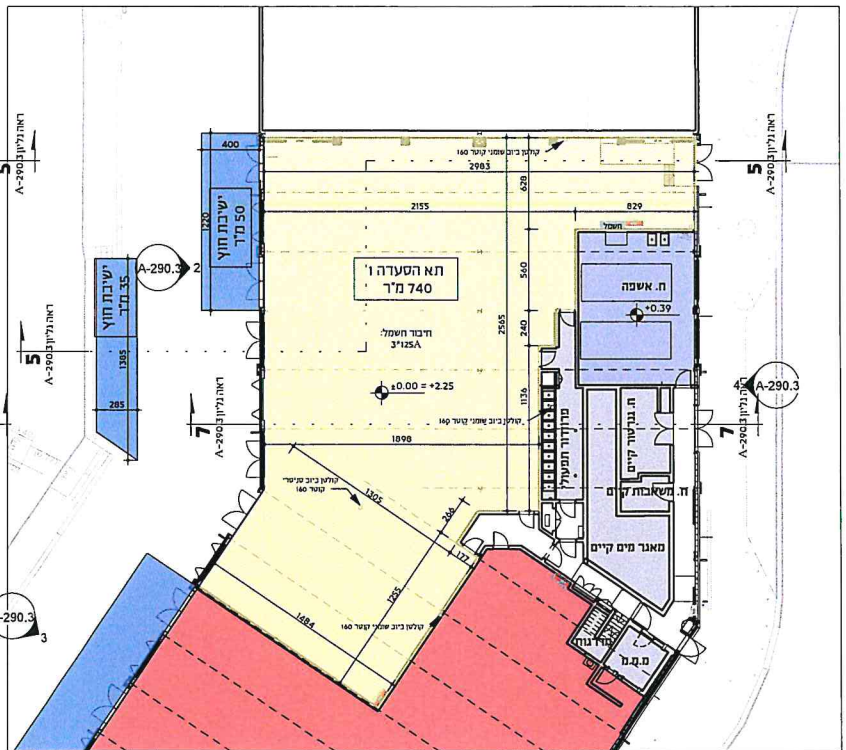
1 תוכנית בר הופעות 1: 250
