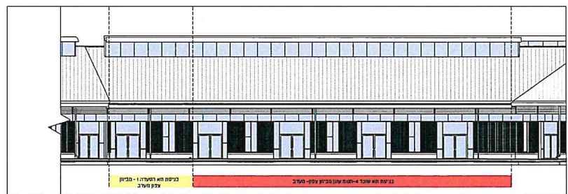
3 חזית צפון מערבית 1: 250
