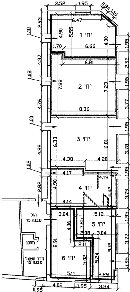
מבנה 15- מלואה קנימ 1:100 מ"ר 30.40
