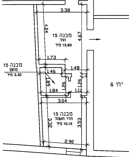
מבנה 15- מלואה קנימ 1:100 מ"ר 30.40
