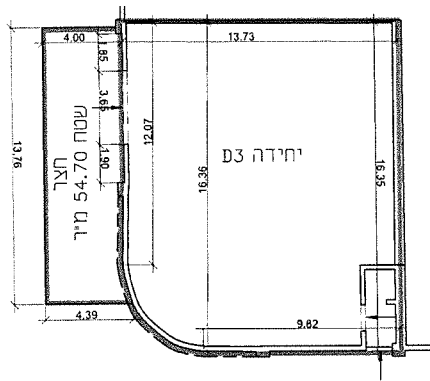
קומת קרקע שטח 220.80 מ"ר (ברוטו)
